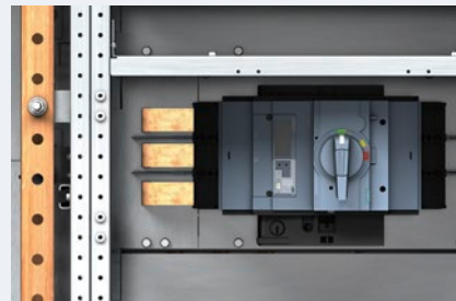
Modulares Gehäuse , optimal abgestimmt auf innovative kommunikationsfähige SENTRON-Komponenten
